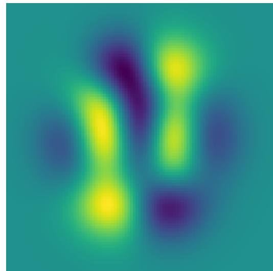
\partial f/\partial y
