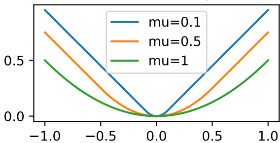
Moreau Envelope
